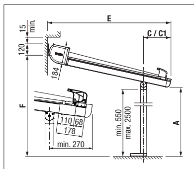
Wandmontage met steunvoet
